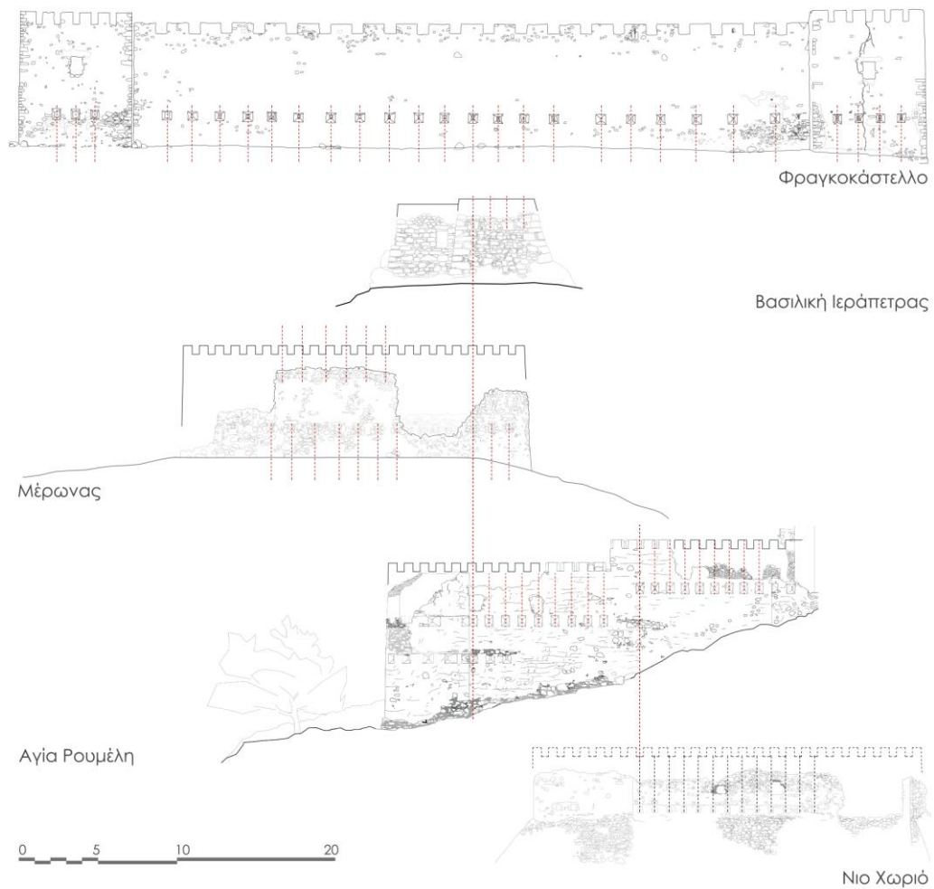
Εικόνα 5. Τυπολογική κατάταξη κουλέδων της Κρήτης σε σχέση με την πυκνότητα των τυφεκιοθυρίδων (σχεδιασμός Μάνος Παπαδάκης).
